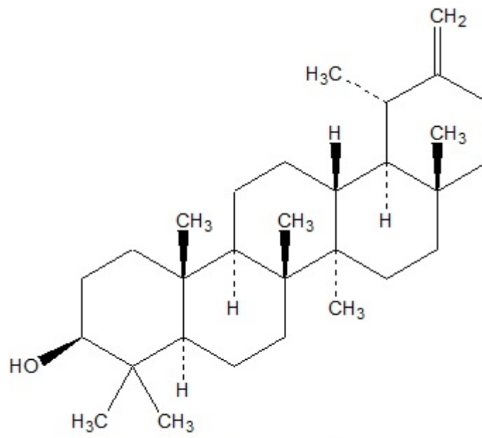
Taraxasterol
